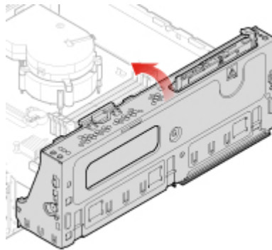
Abbildung 61. Abdeckung der Wi-Fi-Karte (Typ 1 und Typ 2) installieren
