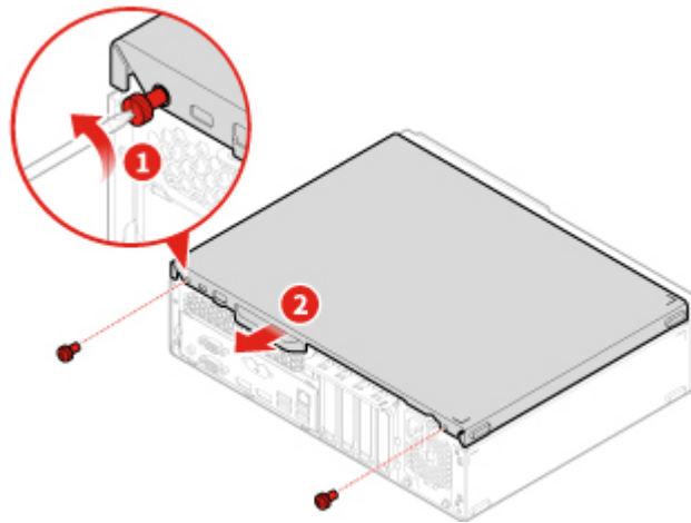
Abbildung 25. Computerabdeckung entfernen
