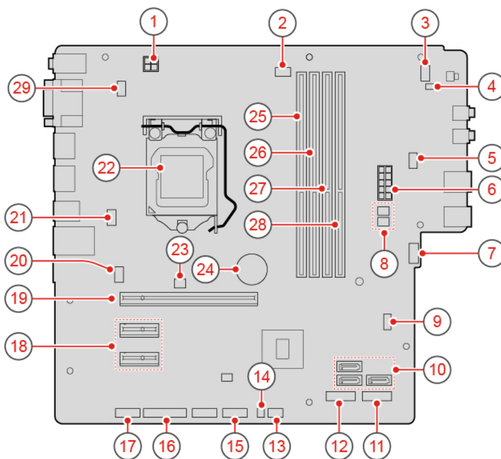
Abbildung 3. Systemplatine
