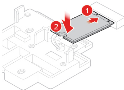
Abbildung 75. M.2-Solid-State-Laufwerk installieren
